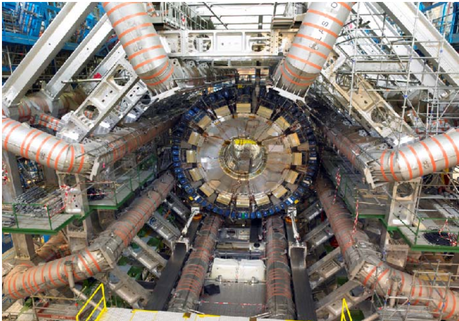
Vista del calorímetro en su posición final, juntamente con los imanes toroidales
