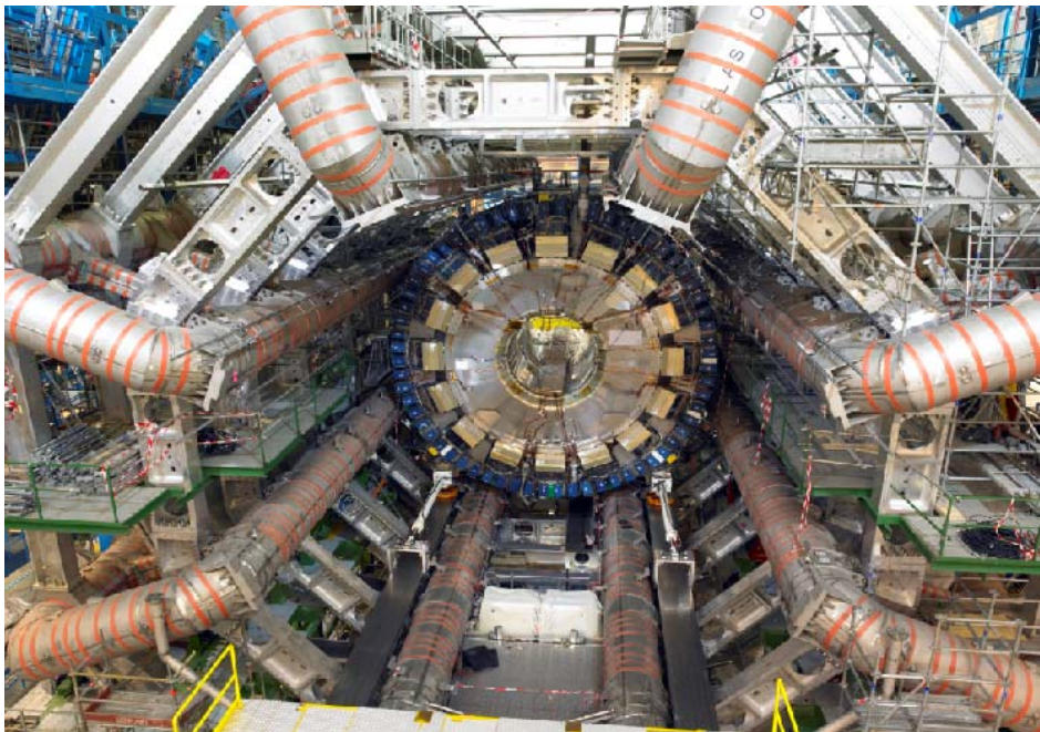
Vista del calorímetre central en la seva posició final, juntament amb els imants toroidals.
