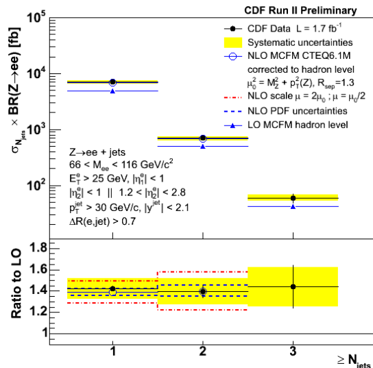
Sección eficaz de producción de sucesos Z+jets
