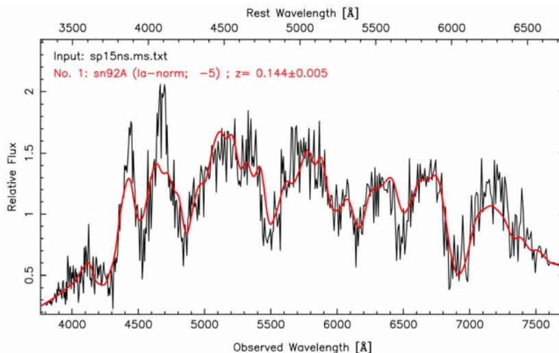
Espectro de la supernova SN2007ph, ( z=0.144 ), obtenido el 5 de Noviembre de 2007 con el TNG. Puede verse superpuesto un espectro de una supernova estándar de tipo Ia, desplazado a z=0.144 , observada cinco días antes del máximo de luz.
