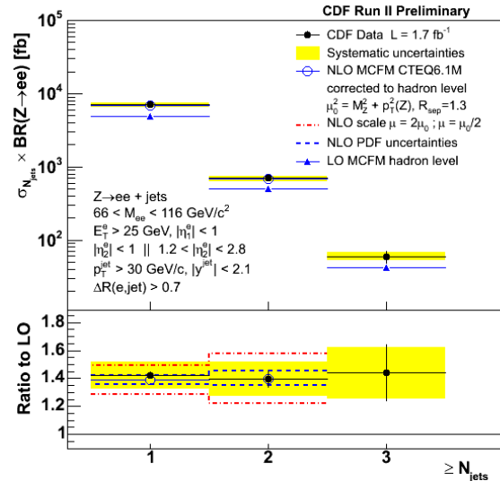
Secció eficaç de producció de successos Z+jets.
