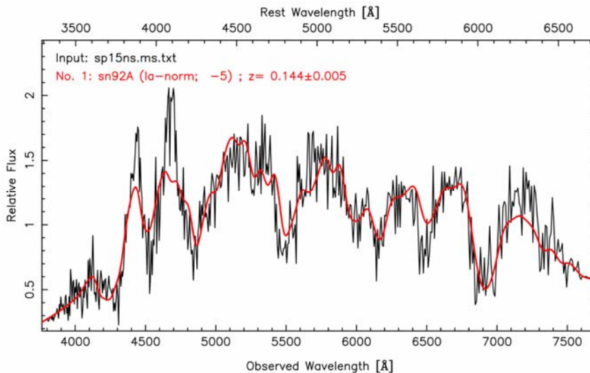
Espectre de la supernova SN2007ph, a un desplaçament al roig de z=0.144 , pres el 5 de novembre de 2007 al TNG. Podem veure superimposat l'espectre d'una supernova estàndard del tipus Ia, desplaçat a z=0.144 , observada cinc dies abans de produir-se la màxima emissió de llum.
