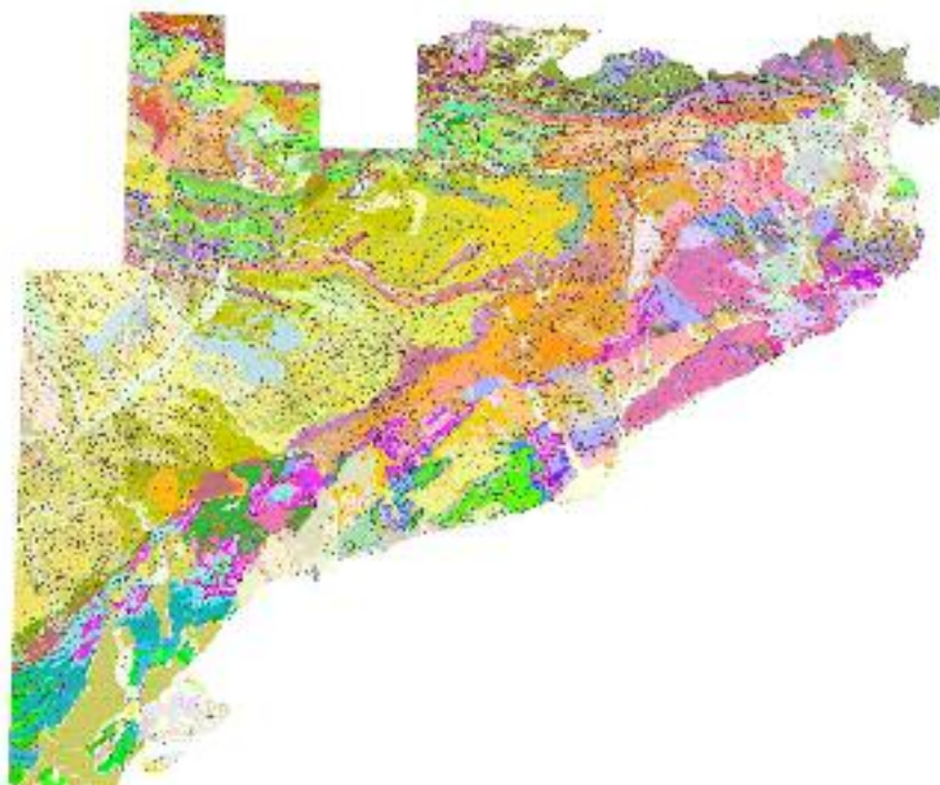
Mapa 2.15. Base de dades geològiques 1:50 000 (Mapa d'estat, juny 2005).
