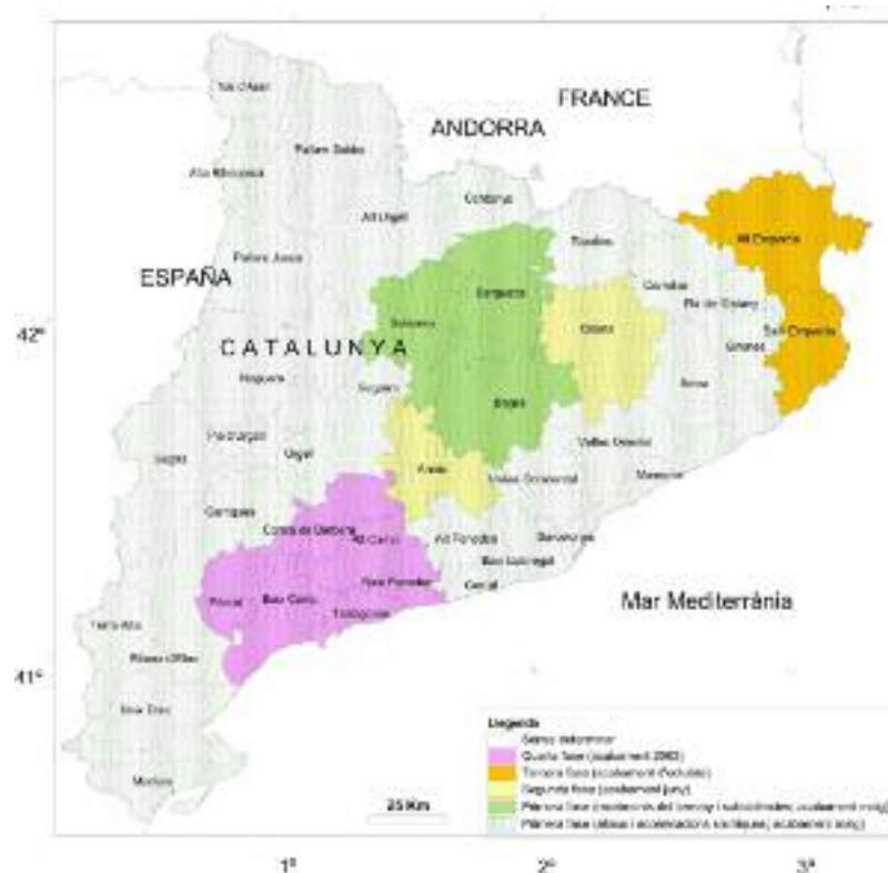
Mapa 2.20. Representació de les comarques cobertes pel mapa de prevenció de riscos geològics. L'estudi de les allaus i l'acceleració sísmica bàsica cobreix tot Catalunya.
