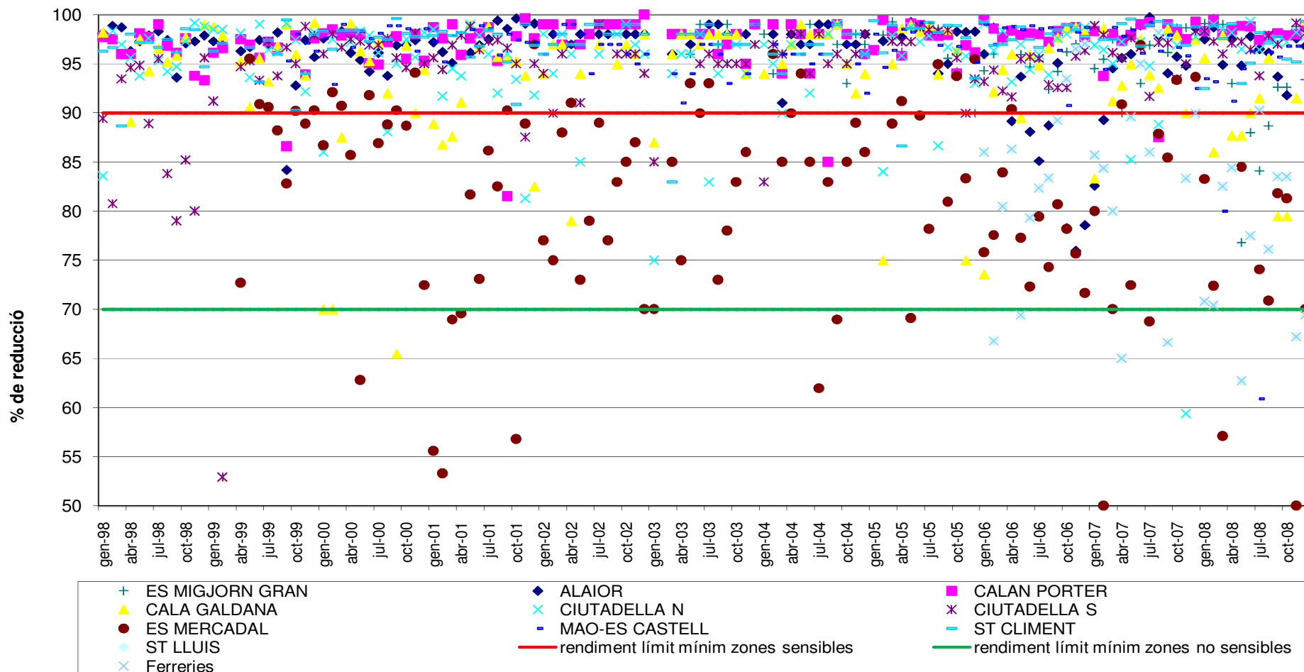
GRÀFIC 2. Rendiment en la eliminació de DBO 5 a les EDARs d'ABAQUA a Menorca. 1998-2008.
