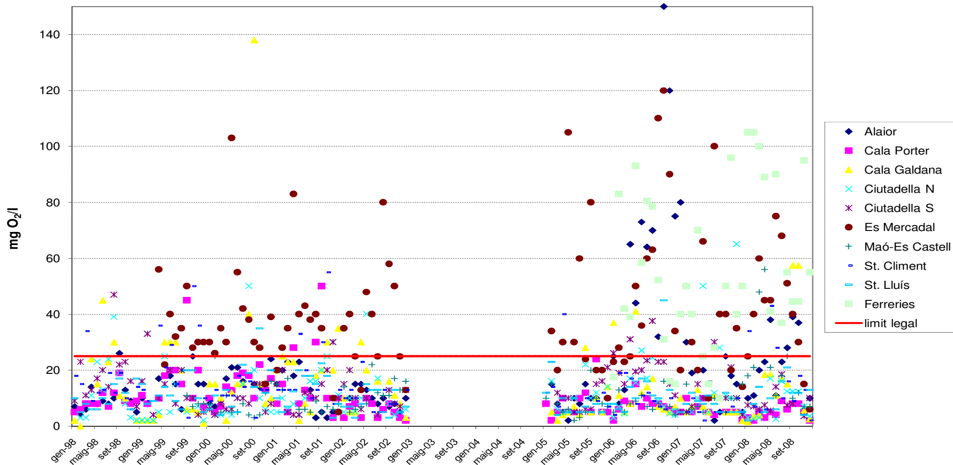
GRÀFIC 1. Valors de DBO 5 a la sortida de les EDARs d'ABAQUA. 1998-2008.
