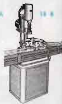
TIPO "ESTRELLA" con plato revolver 28000 botellas jornada.
