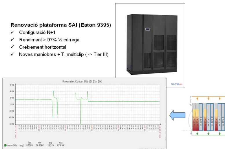
Figura 26. Infraestructura SAI
