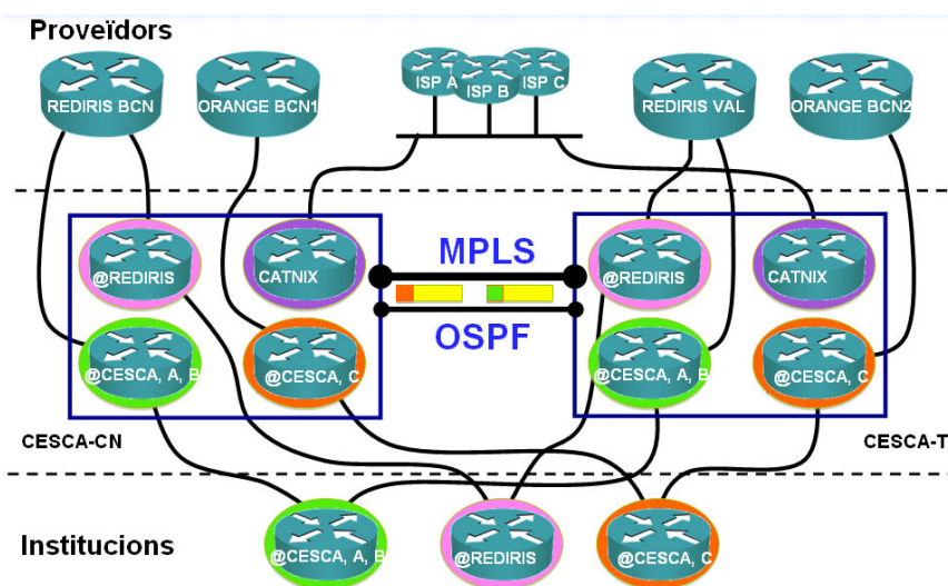
Figura 52. Arquitectura lògica
