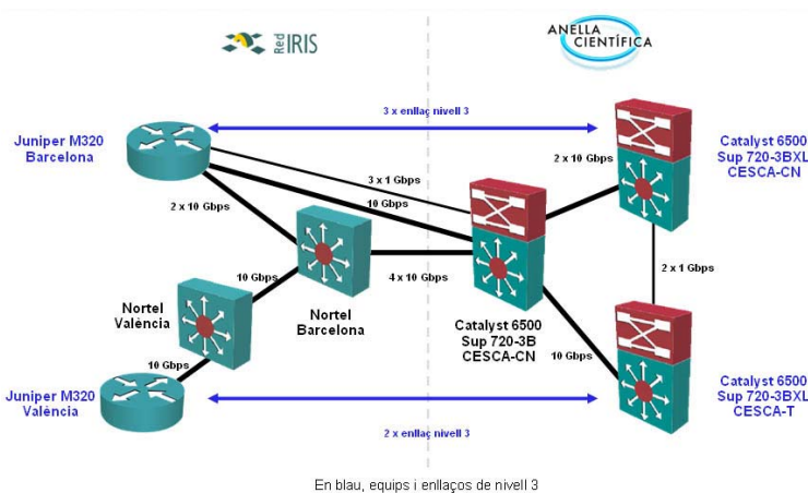
Figura 83. Interconnexió de l'Anella Científica amb RedIRIS
