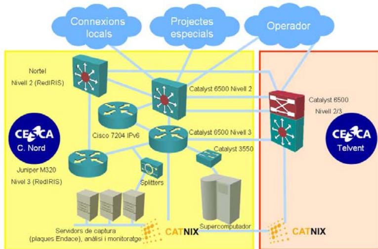
Figura 54. Topologia CESCO
