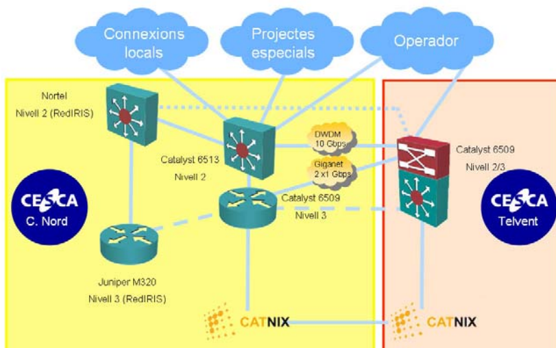
Figura 57. Topologia final
